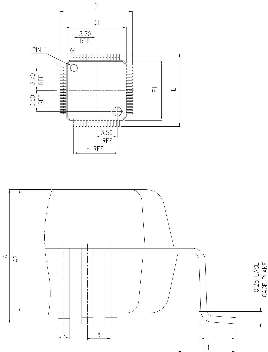
图 14 LQFP64 封装图
