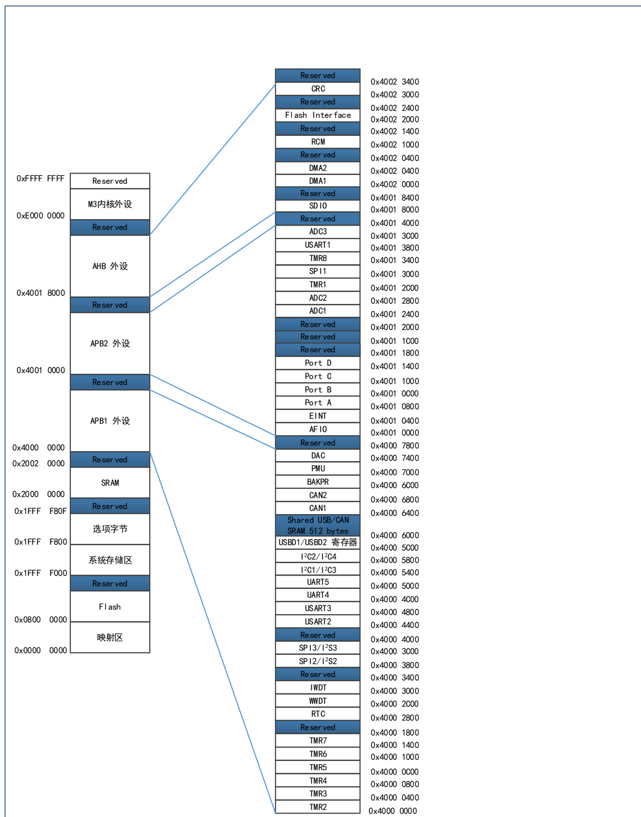
图 3 APM32A103RCTx 型号地址映射图
