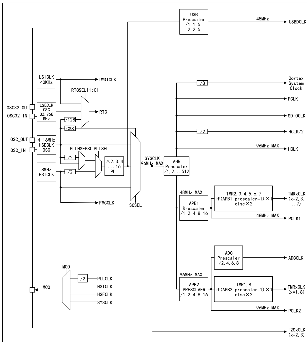
图 4 APM32A103RCTx 时钟树
