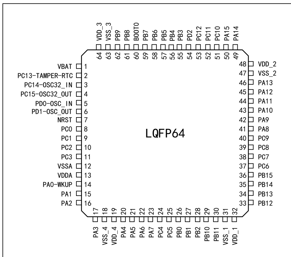
图 1 APM32A103RCTx 型号 LQFP64 引脚分布图
