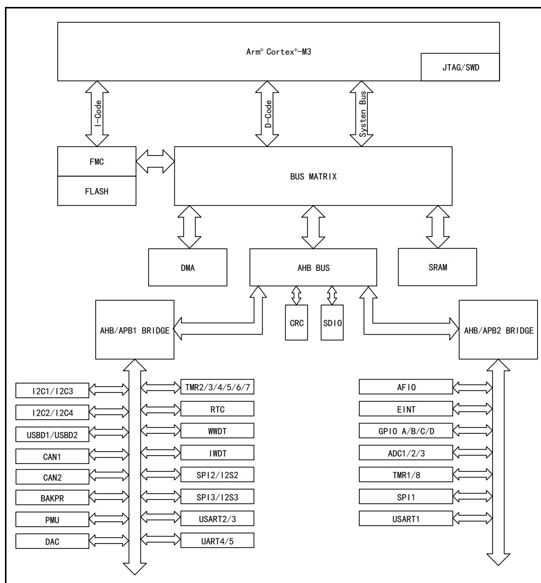
图 2 APM32A103RCTx 系统框图
