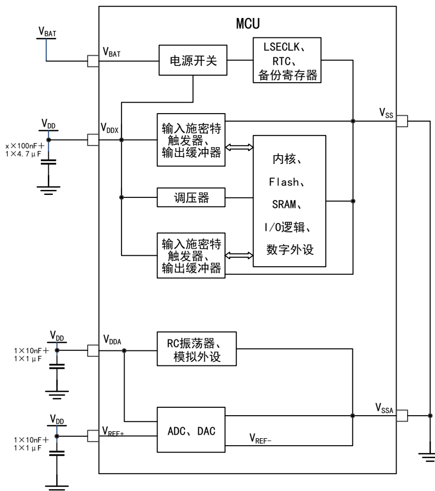
图 5 电源方案
